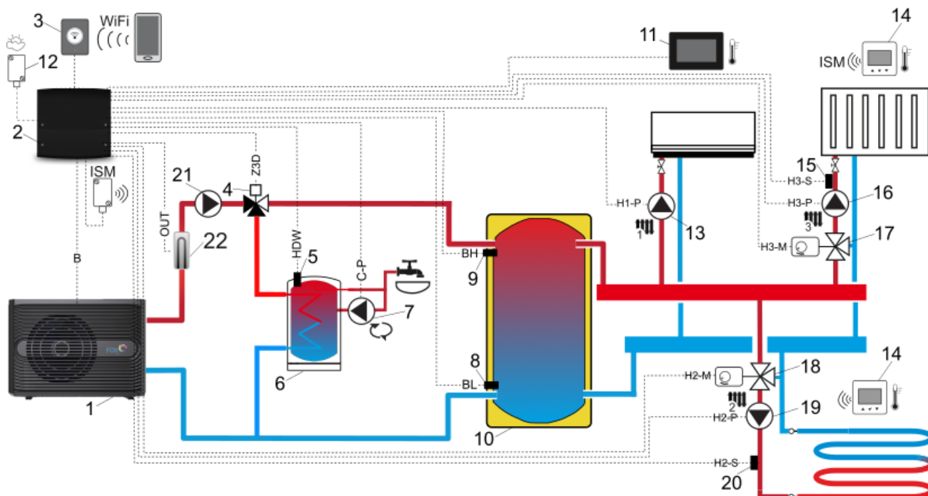
Schemat z buforem ciepła i zasobnikiem CWU 3 (funkcja chłodzenia): 1 – pompa ciepła, 2 – regulator, 3 – moduł internetowy, 4 – zawór 3-drogowy, 5 – czujnik temp. zasobnika CWU, 6 – zasobnik CWU, 7 – pompa cyrkulacji, 8 – dolny czujnik temp. bufora, 9 – górny czujnik temp. bufora, 10 – bufor ciepła, 11 – panel sterujący z funkcją termostatu pokojowego, 12 – czujnik temp. zewnętrznej (pogodowej), 13 - pompa mieszacza 1, 14 – bezprzewodowy termostat pokojowy, 15 – czujnik temp. mieszacza 3, 16 – pomp mieszacza 3, 17 – siłownik mieszacza 3, 18 – siłownik mieszacza 2, 19 – pompa mieszacza 2, 20 – czujnik temp. mieszacza 2, 21 – pompa CWU, 22 – grzałka przepływowa.
